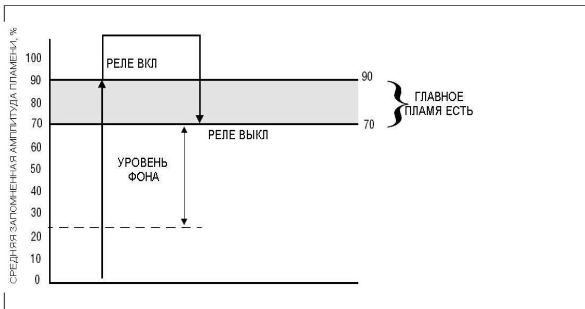
РИСУНОК 11 Пример установки порогов срабатывания реле пламени после изучения фонового пламени
