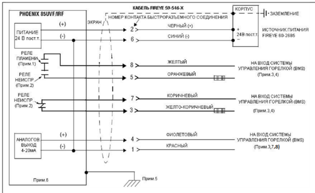
РИСУНОК 7 СХЕМА ЭЛЕКТРИЧЕСКИХ ПОДКЛЮЧЕНИЙ СКАНЕРА
