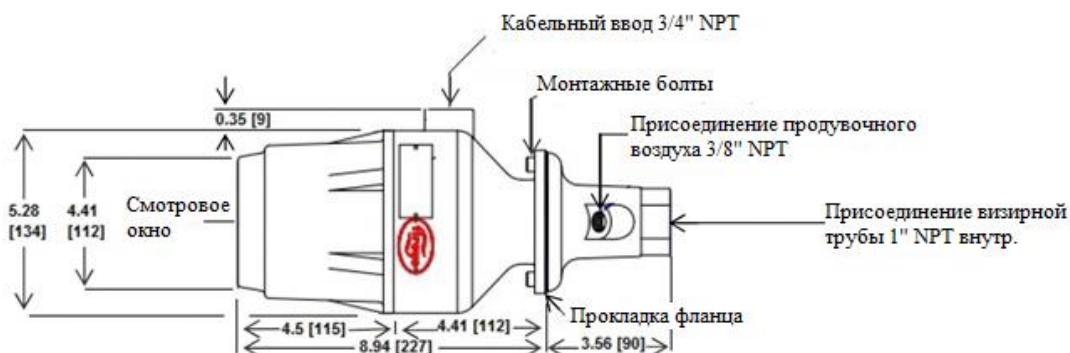
РИСУНОК 2. Сканер Phoenix в корпусе АTEX для опасной зоны (комплект с монтажным фланцем заказывается отдельно)
