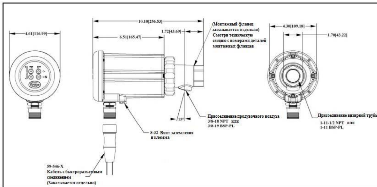
РИСУНОК 1 - Размеры
