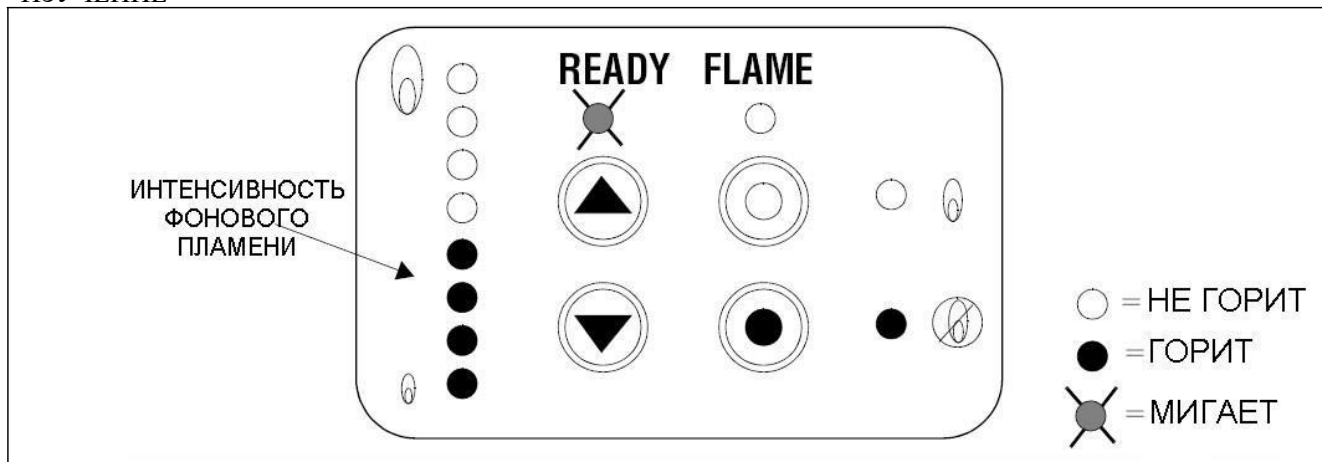
РИСУНОК 11 Пример установки порогов срабатывания реле пламени после изучения фонового пламени
