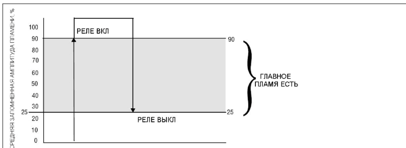
РИСУНОК 10. Пример установки порогов срабатывания реле пламени (в режиме изучения только главного пламени)
